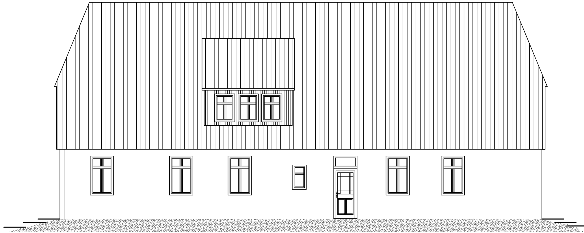
West-Ansicht
